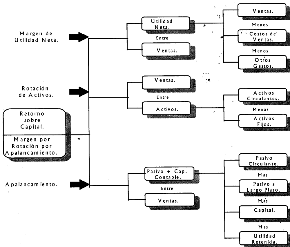
Fig. 8 Modelo Dupont.
